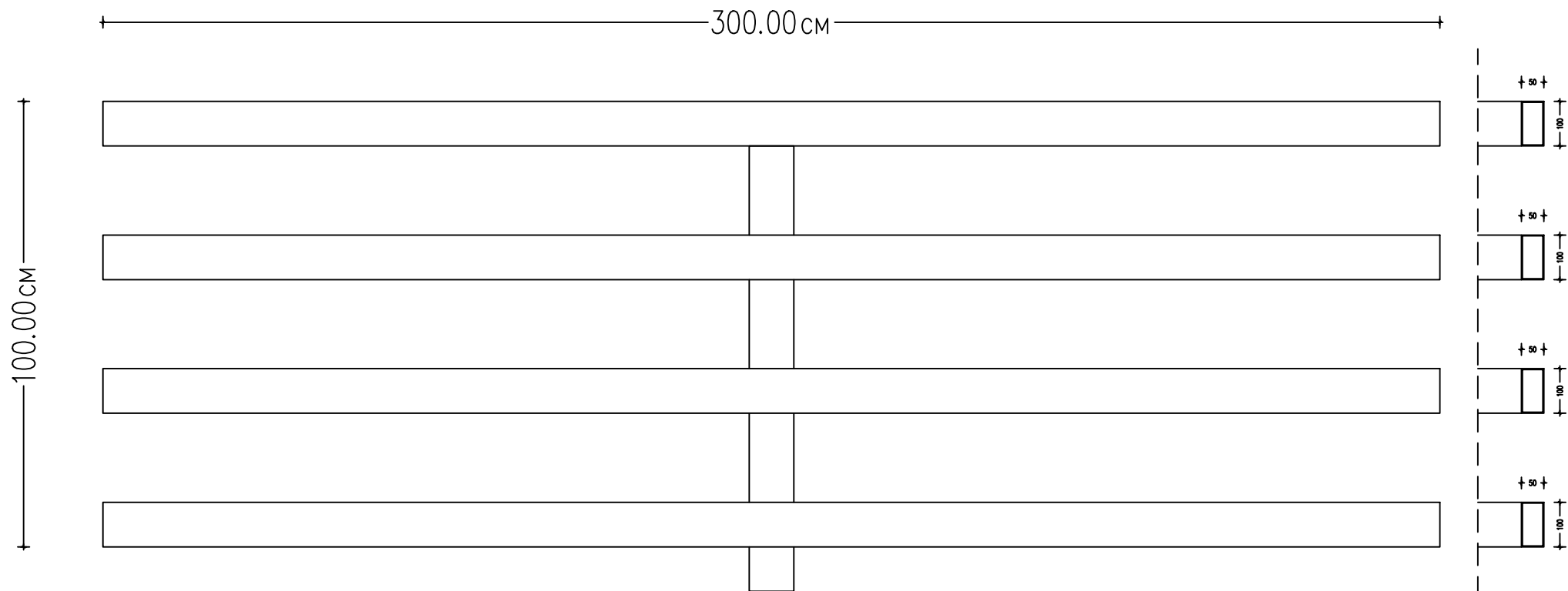
Парапет за прозорци от неръждаема стомана с профил 100/50/3
